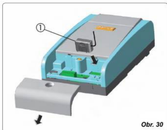
12.1. Uložení radiových ovladačů 868 do paměti
